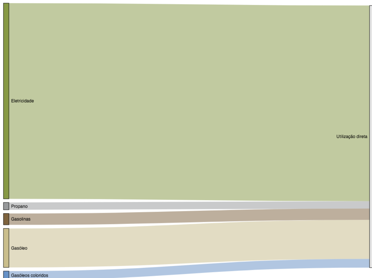
Figura 36: Diagrama de Sankey da utilização de fontes de energia primária no Município de Fronteira
